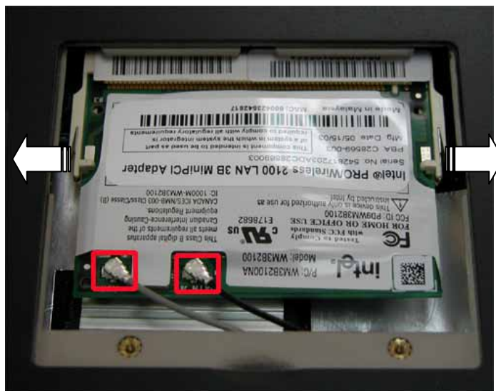
Fig. 9 Wireless LAN & MCD Modem Module
